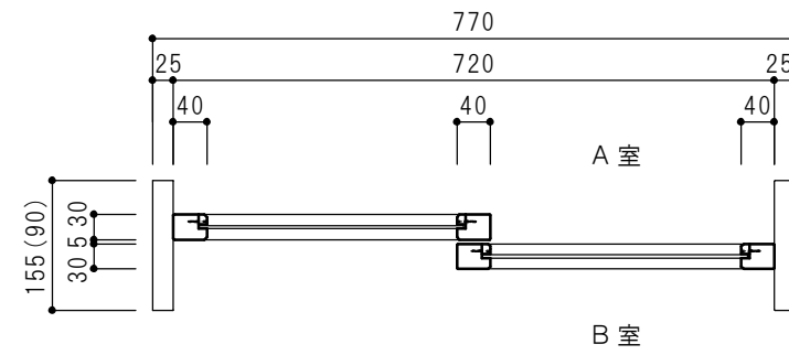
ヨコ断面図
