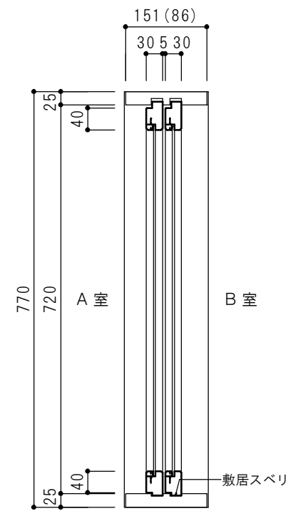
タテ断面図
