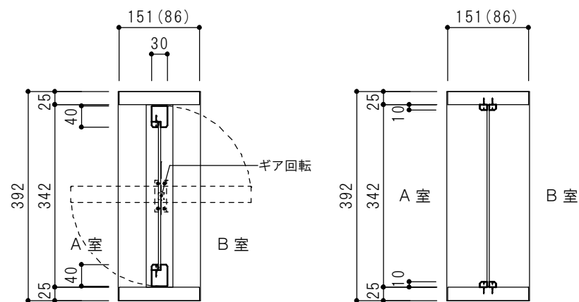
タテ断面図 横軸回転窓
