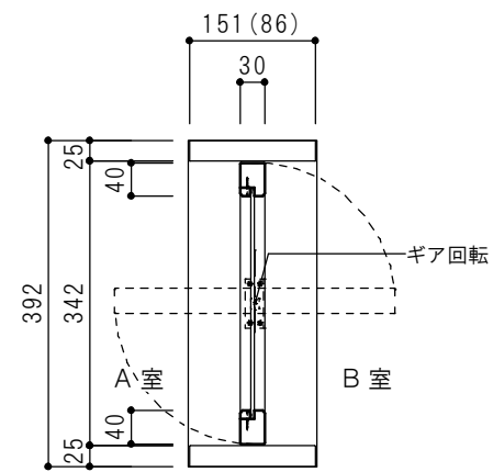
タテ断面図
