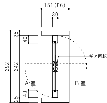
タテ断面図
